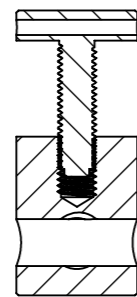
SECTION A-A SCALE 1 : 1
