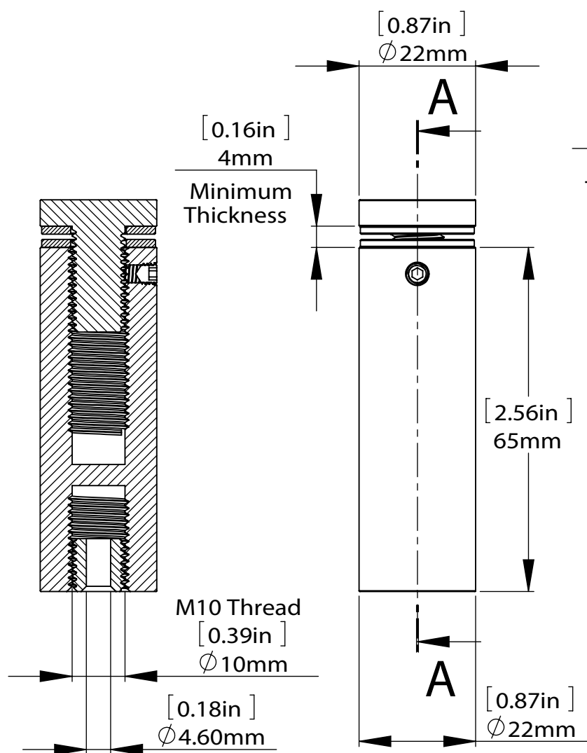
SECTION A-A
