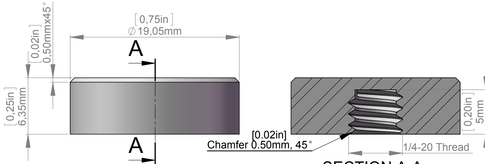
SECTION A-A SCALE 4 : 1
